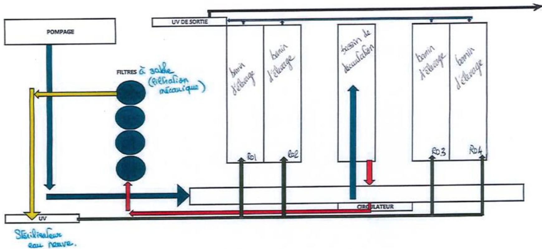
Annexe 2 : Schéma du circuit fermé avec la station de traitement en entrée
