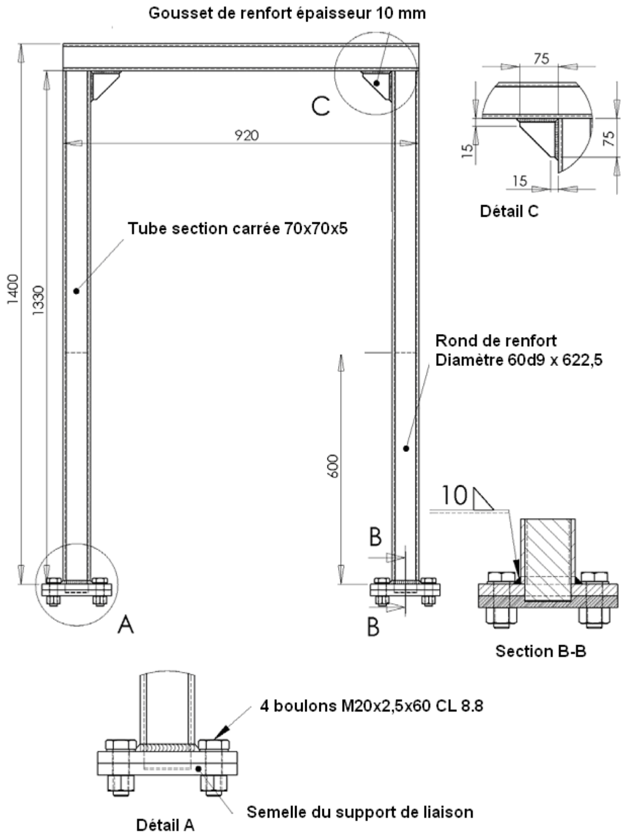
Figure 1. Arceau arrière fixe
