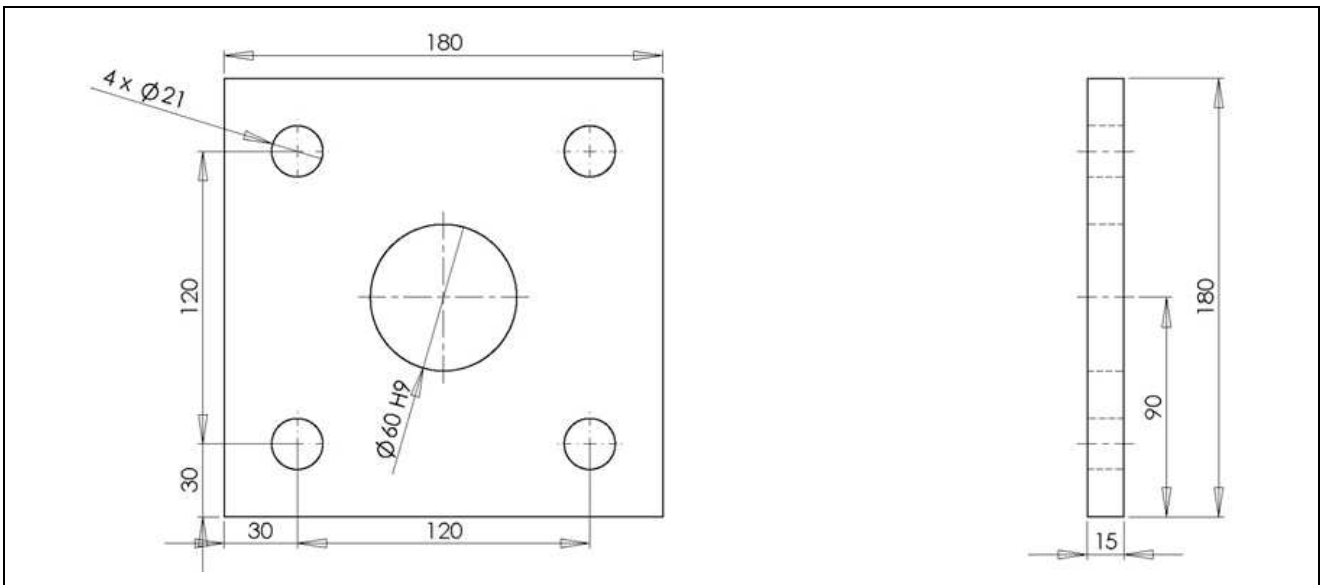
Figure 2. Semelle (base de montants verticaux)
