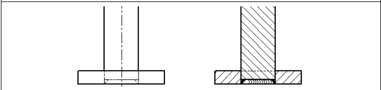
Figure 3. Soudure des ronds de renfort
