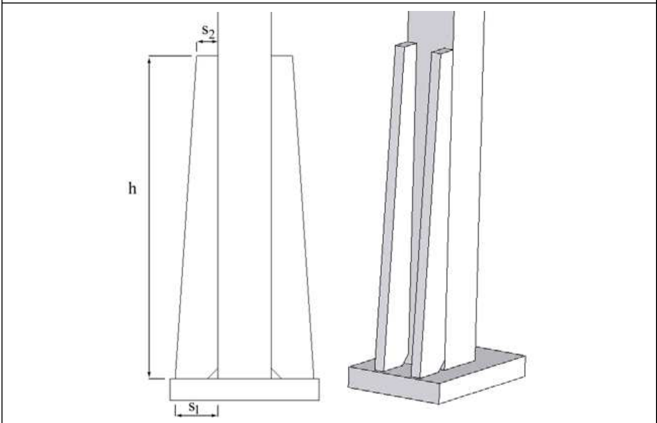
Figure 4: Gousset de renfort
