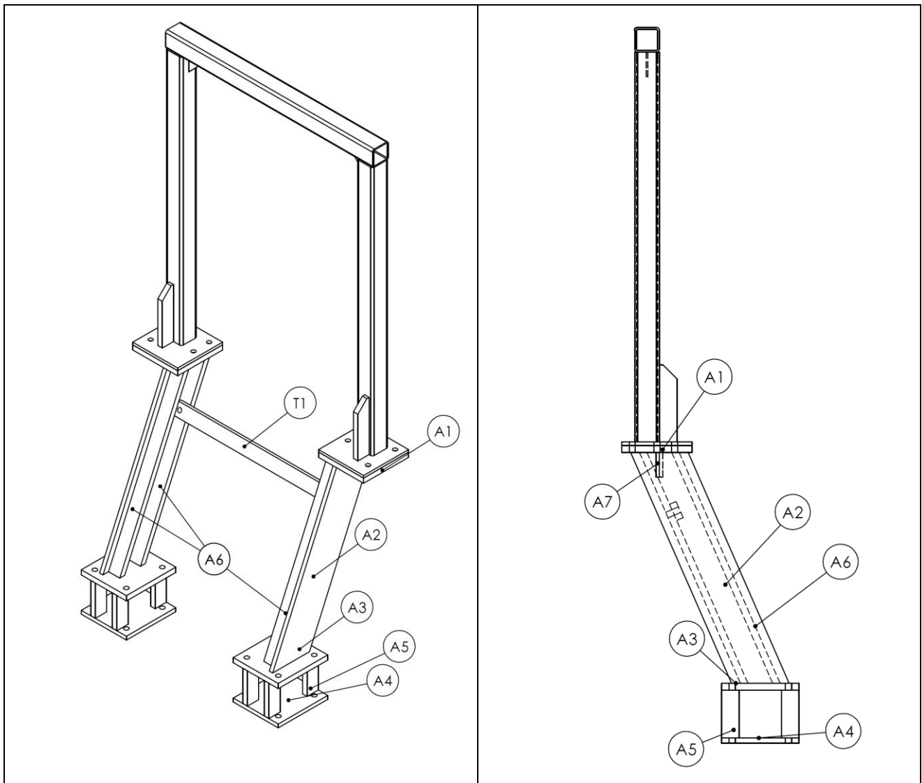
Figure 1. Structure de protection en cas de renversement à deux montants arrière pour tracteur à roues SAME D.A. 30
