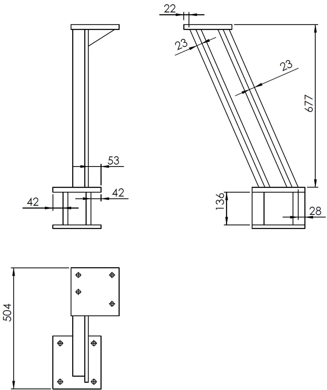
Figure 2. Cotes d'assemblage et plans de réalisation
