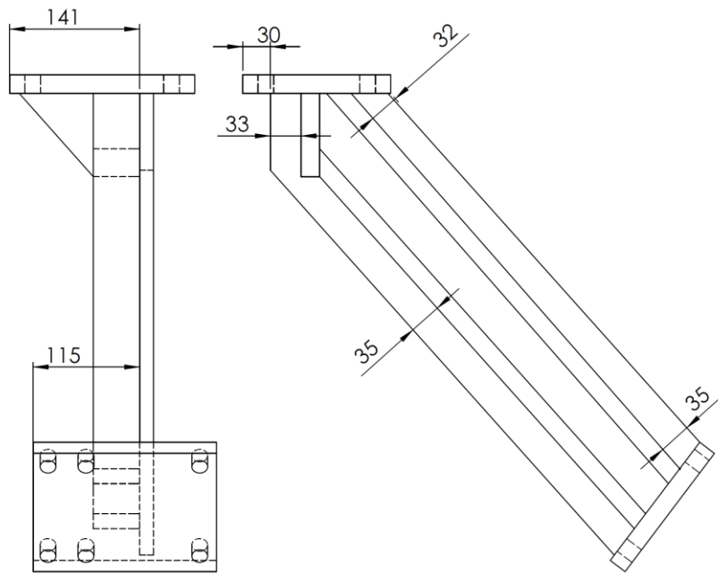
Figure 2. Cotes d'assemblage et plans de réalisation
