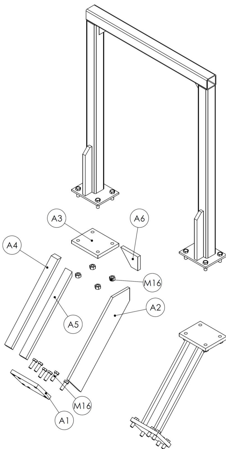
Figure 1. Structure de protection en cas de renversement à deux montants arrière pour tracteur à chenilles FIAT 351C et similaires
