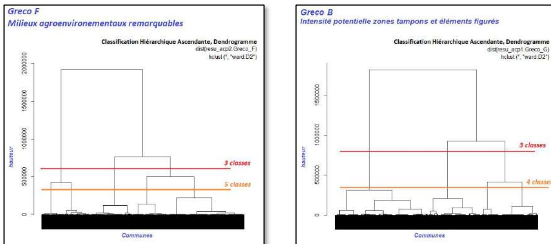
Figure 3-3-6 : exemples de classification hiérarchique ascendante des communes pour 2 régions Greco et 2 familles d'indicateurs. Représentation graphique sous la forme d'un dendrogramme, qui permet de choisir un nombre de classes opportun ; via la « hauteur » (axe des ordonnées) à laquelle on désire « couper » (horizontalement) le dendrogramme (3 ou 5 classes par exemple sur le graphe de gauche, 3 ou 4 classes par exemple sur le graphe de droite ; même si dans les deux cas 2 grands groupes distincts apparaissent). Ces classes fourniront les centres d'intérêt pour la classification via les « nuées dynamiques » (regroupement des communes autour de ces centres, « noyaux »).
