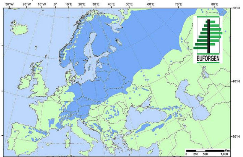
Aire de distribution naturelle du pin sylvestre en Eurasie (EUFORGEN 2008)
