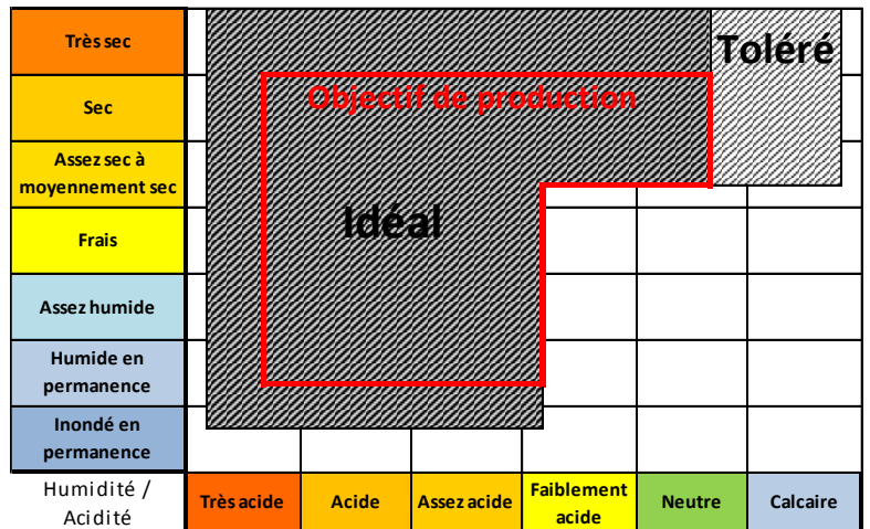
Diagramme des conditions pédologiques favorables, en eau et en pH (zones grisées) et des conditions pédologiques retenues pour un objectif de production (en rouge)
