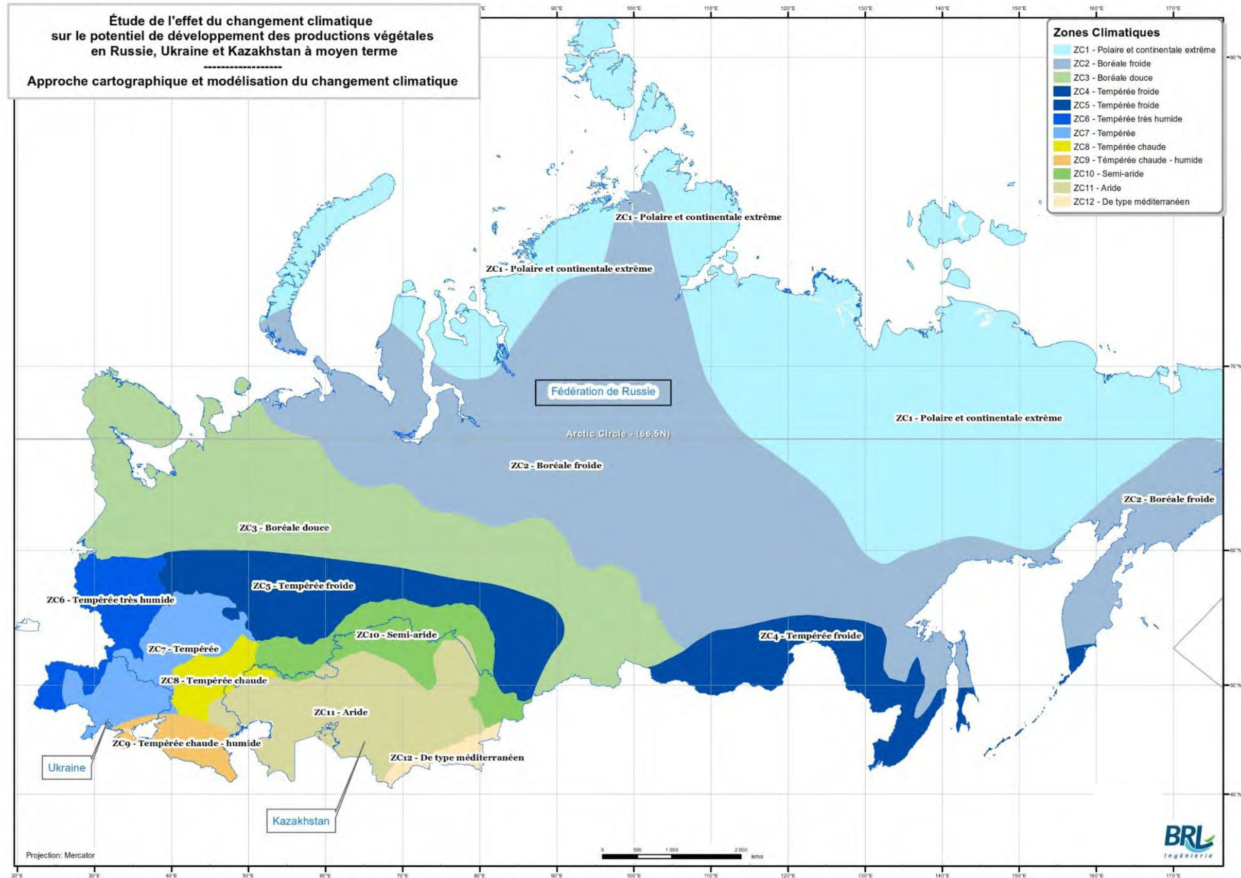
Figure 16 : Zones climatiques
